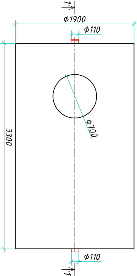
Вид сверху
