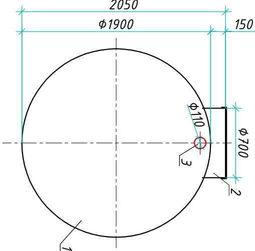
Вид А
